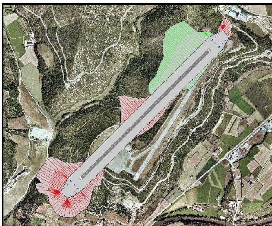
Figura 56. Encaix de l'alternativa A1 (terraplenat en vermell i desmunt en verd) Font: INYPSA
